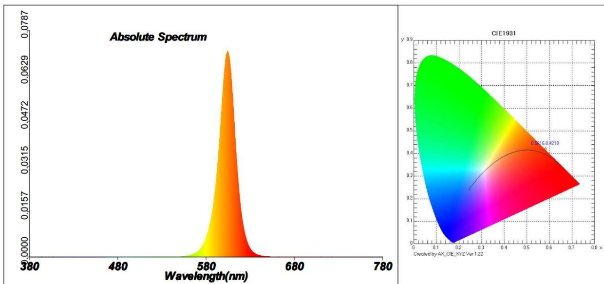
Спектр Свечения
