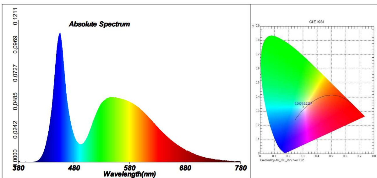
Спектр Свечения
